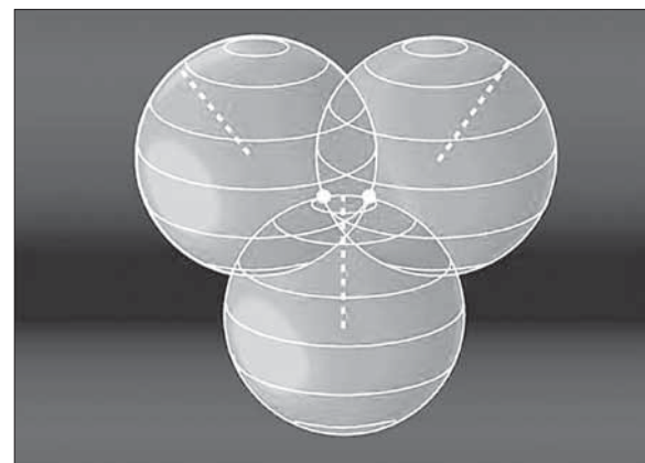
Три сферы пересекаются только в двух точках пространства
